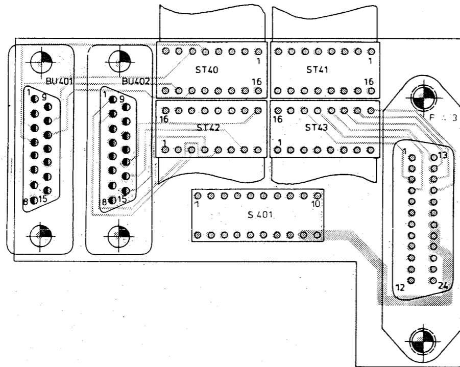
Ansicht und Leitungsführung Bauteilseite (Innenlage DV12) View of tracks on component side
