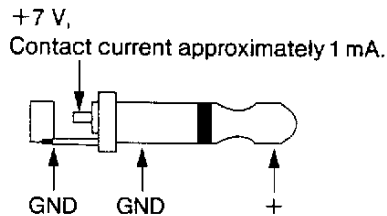
Plug wiring
